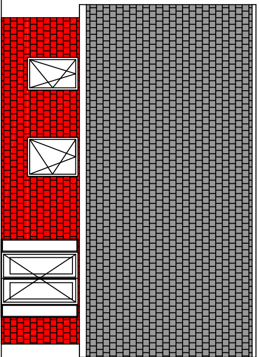
Achter aanzicht
